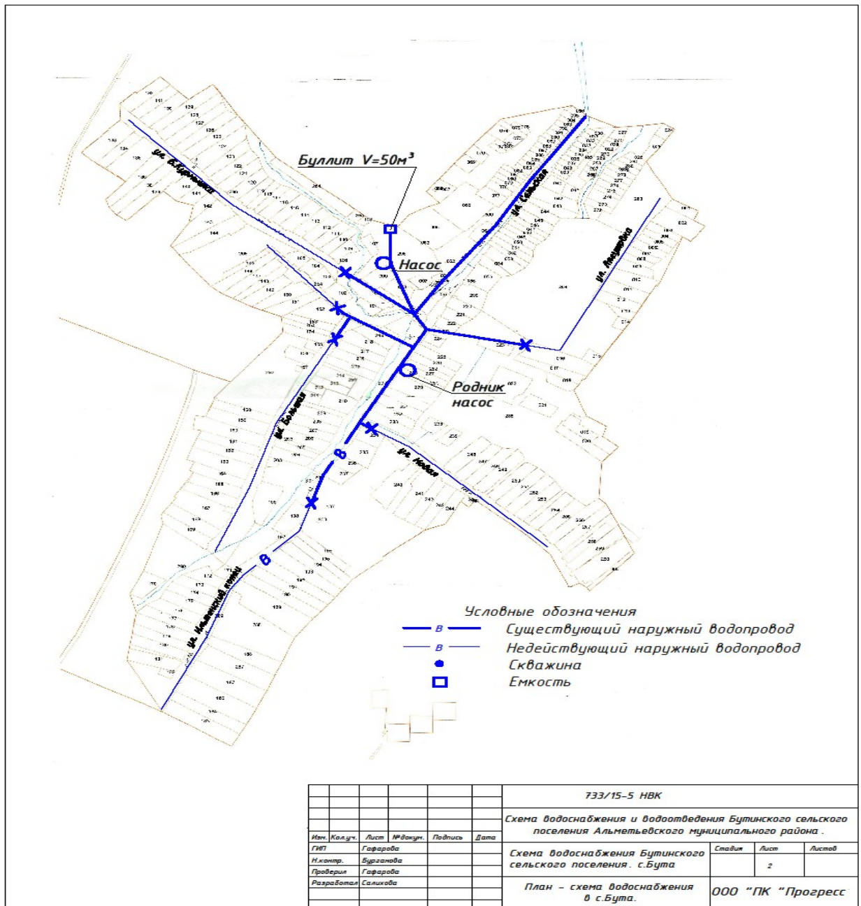
Рис. № 1 Схема водоснабжения
